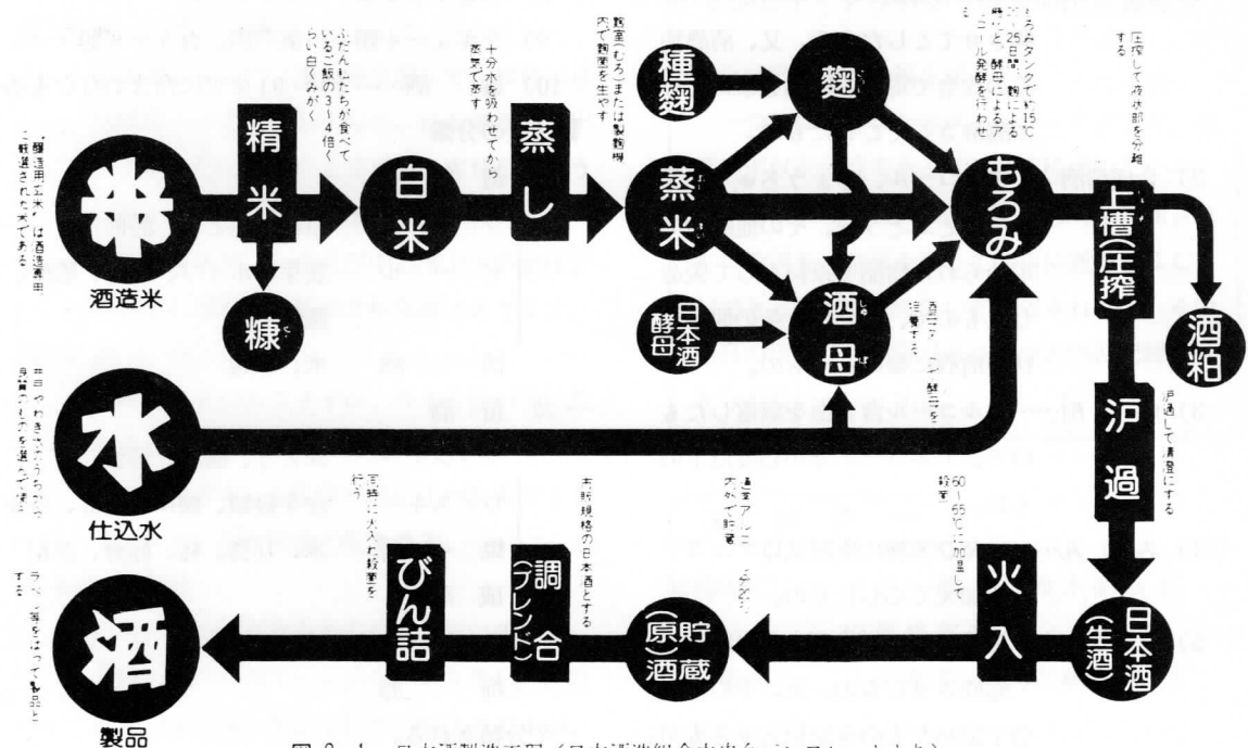
図 2-1 日本酒製造工程 (日本酒造組合中央会パンフレットより)
